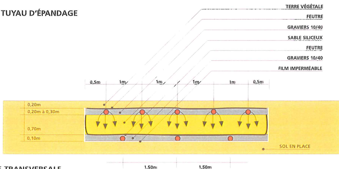
COUPE TRANSVERSALE
