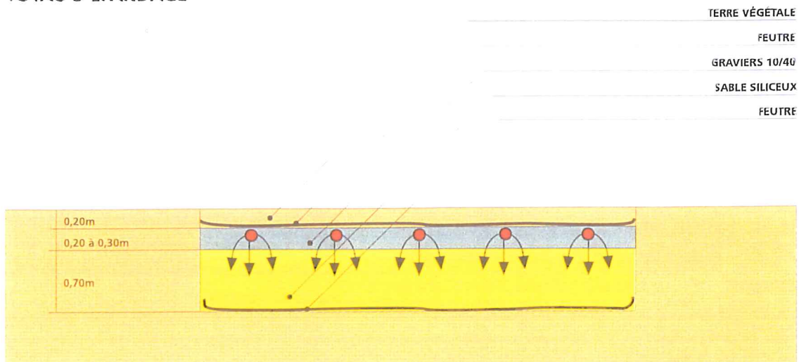
TUYAU D'ÉPANDAGE
